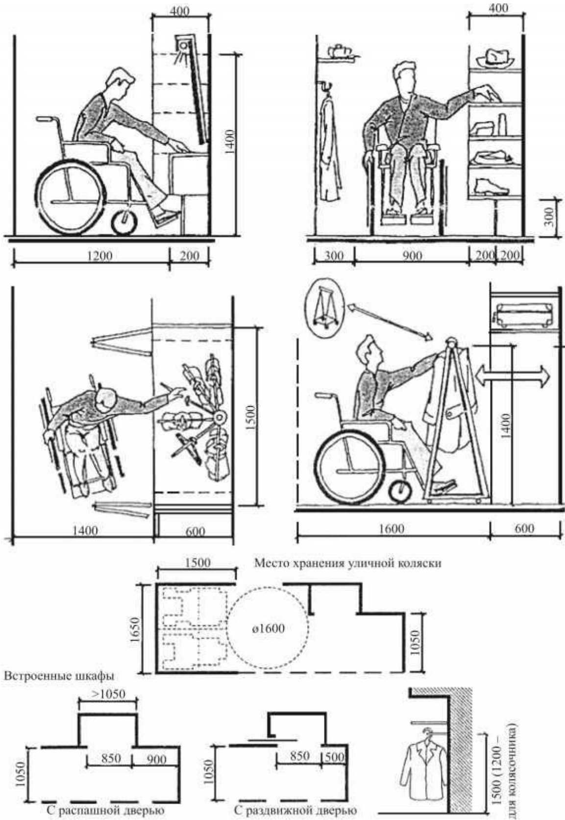
Рисунок А.7 – Оборудование передней
